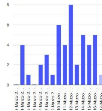
Explosión
