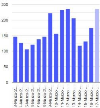
Exhalaciones
